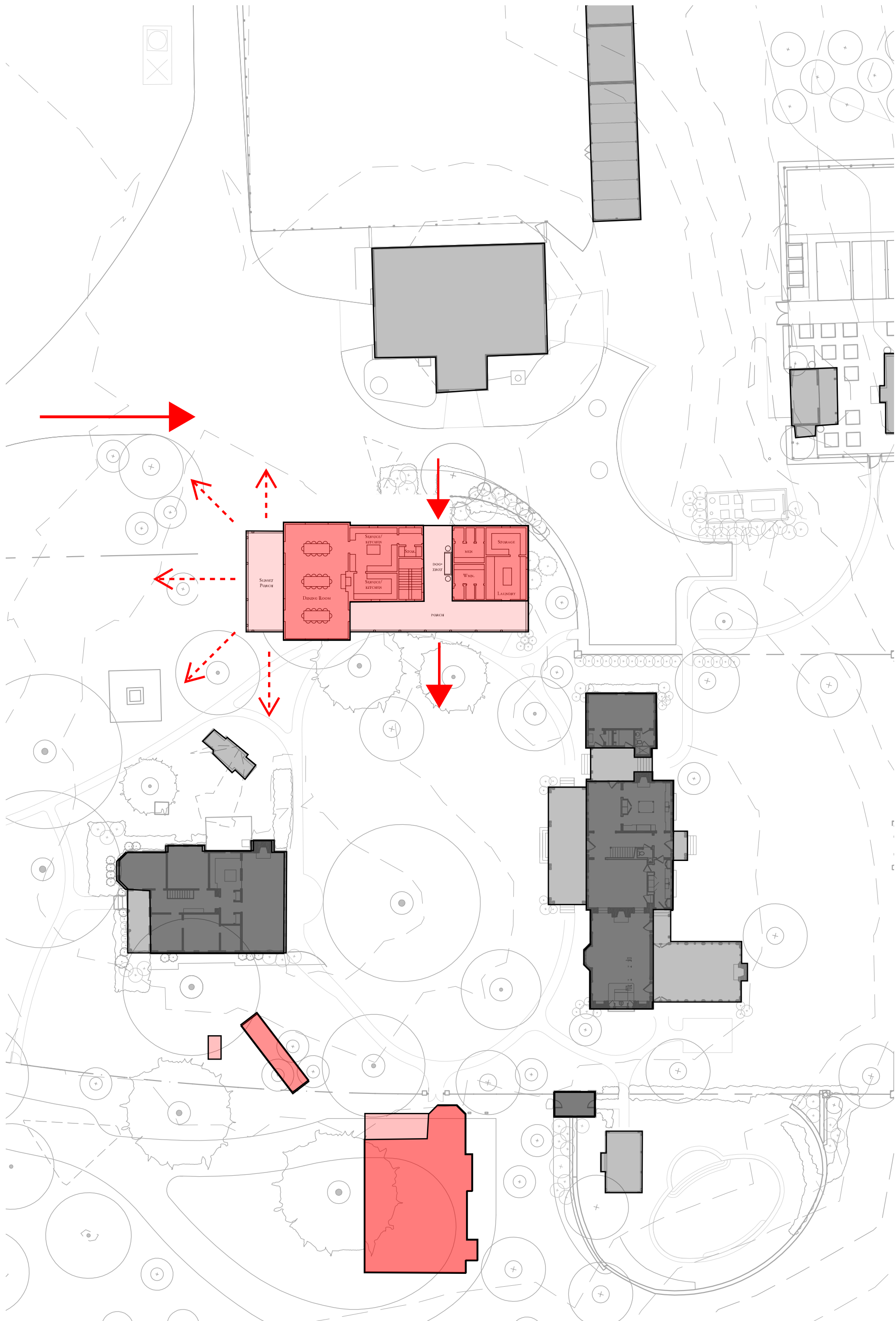
OPTION 1 SITE PLAN
